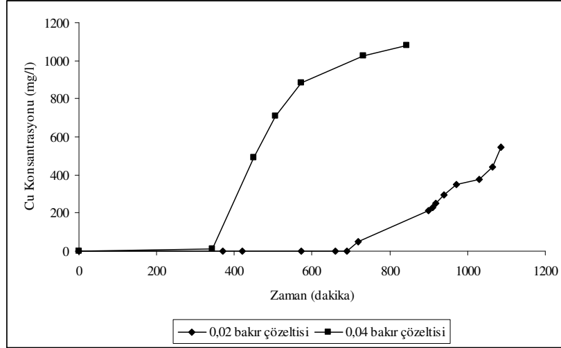
Şekil 1. 0,02 N ve 0,04 N sentetik bakır çözeltisi kolon çıkış suyundaki bakır konsantrasyonunun zamanla değişimi
